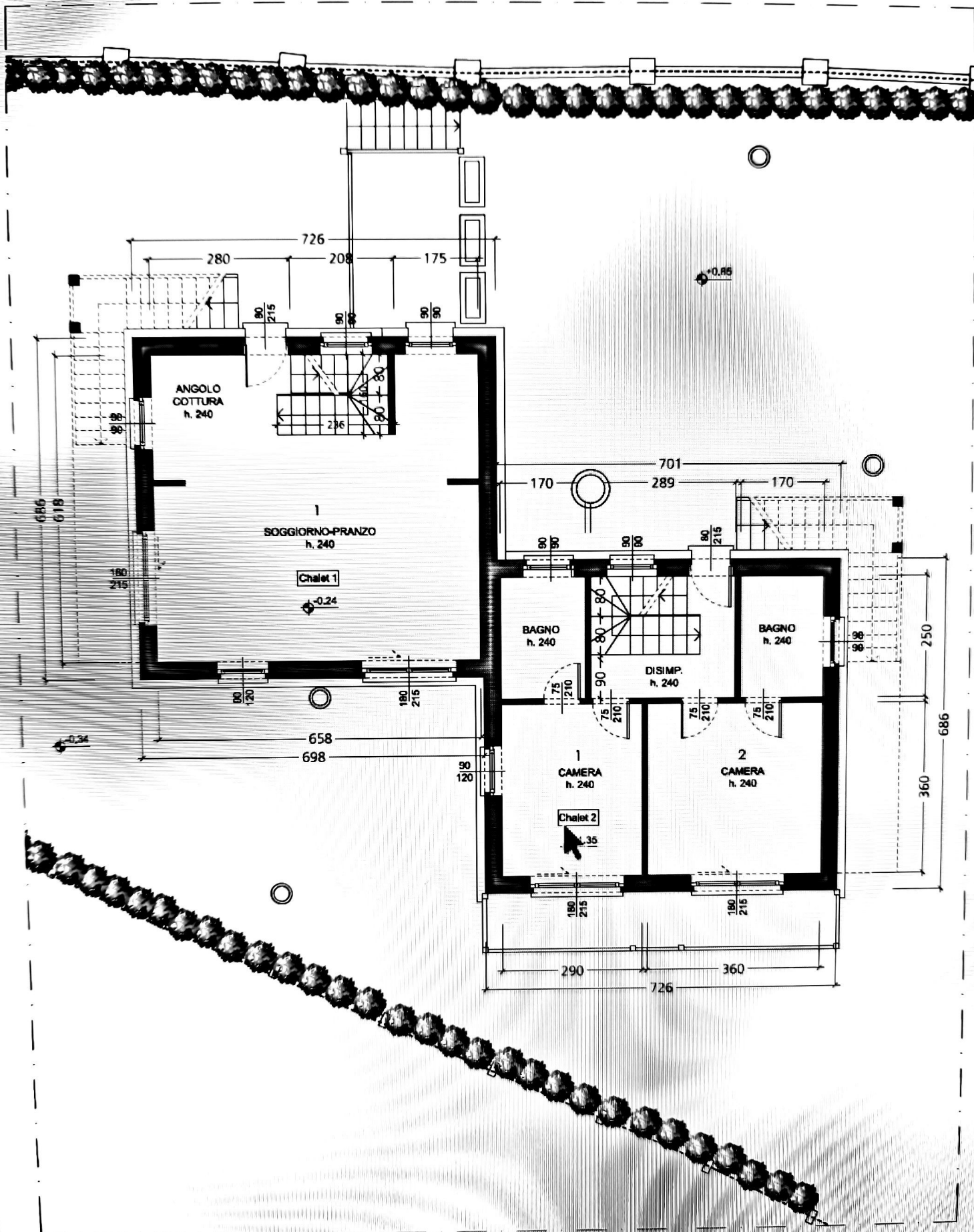
PLANIMETRIA PIANO TERRA STATO DI PROGETTO
